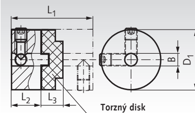
Zaistovacia skrutka
