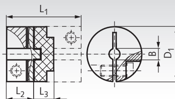
Upínacie
