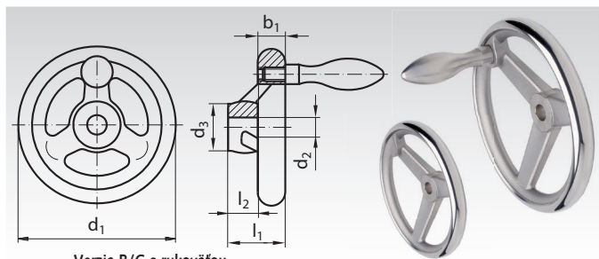
Verzia B/G s rukoväťou
