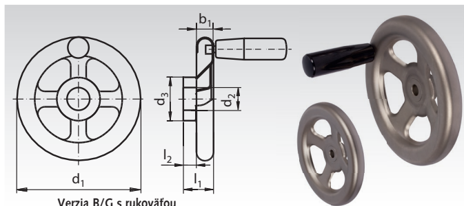
Verzia B/G s rukoväťou
