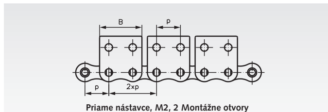
Priame nástavce, M2, 2 Montážne otvory
