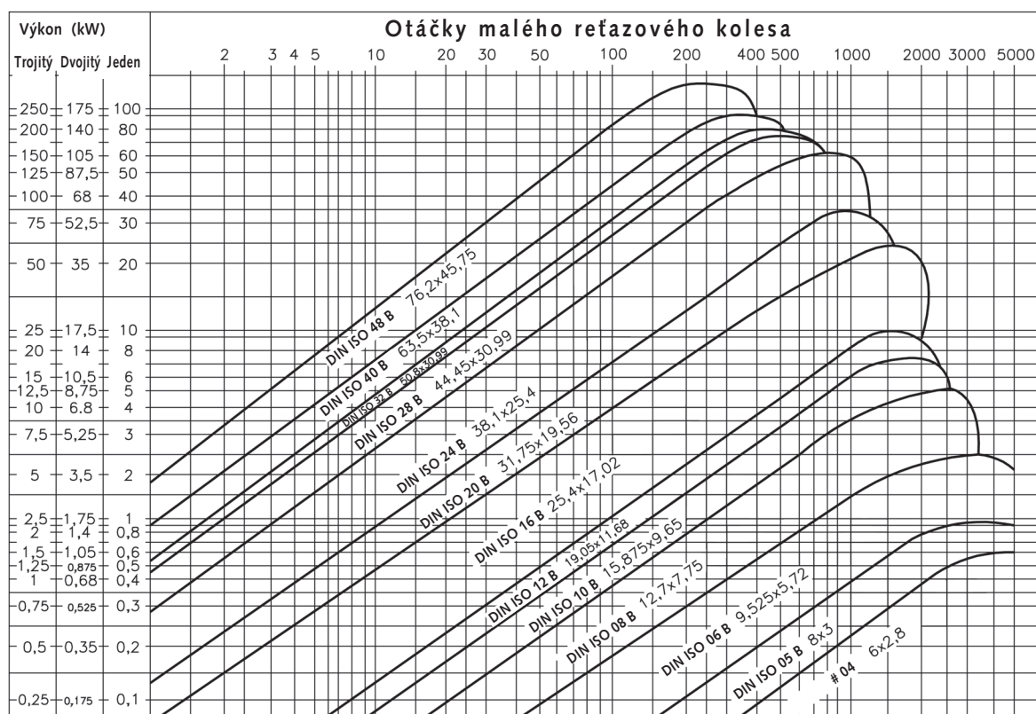
Diagram výkonu: Výpočet výkonu P_B
