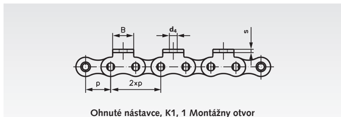
Ohnuté nástavce, K1, 1 Montážny otvor
