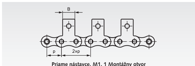
Priame nástavce, M1, 1 Montážny otvor
